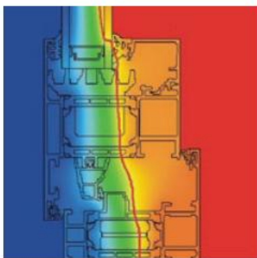
Óptimo isolamento térmico com junta central
