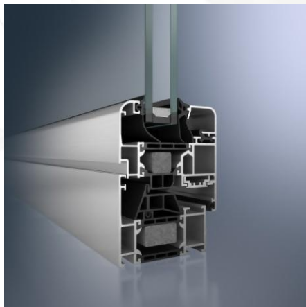
Fenêtre Schüco AWS 70 SL.HI (Soft Line)
