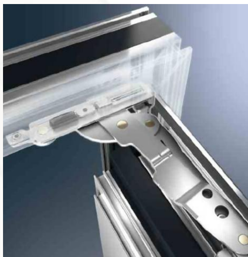
Schüco AvanTec montage amélioré
